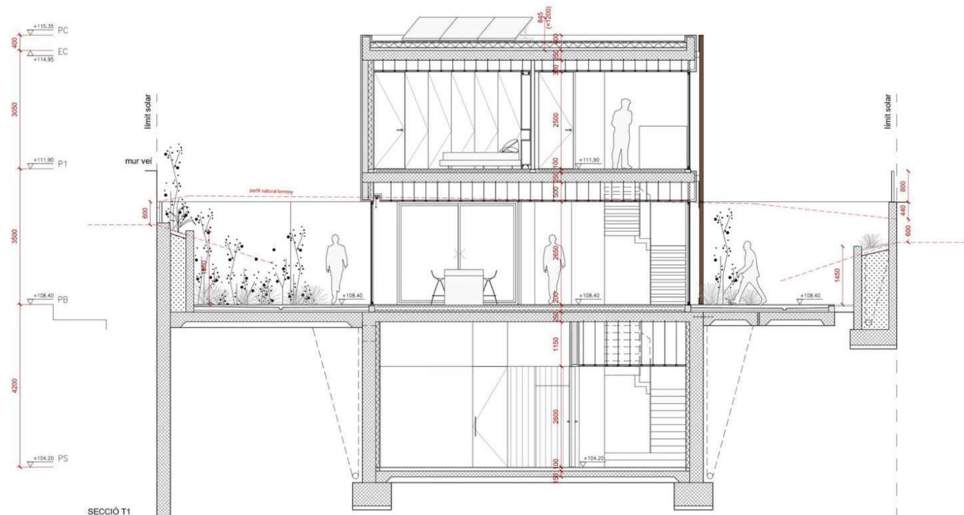
SECCIÓ T1
